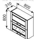
MS 1 Modul superior cu (vitrină)
