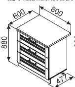
MI 1 Modul inferior cu 3 sertare
