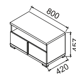
Comoda TV 0,8m
