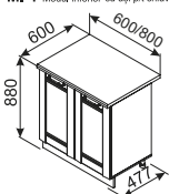
MI 4 Modul inferior cu uși și pîi chiuveță
