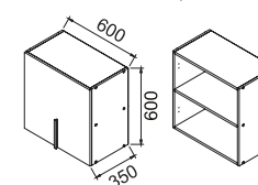
Suspendat cu ușă 0,6m
