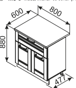
MI 5 Modul inferior cu sertar și uși
