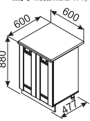
MI 3 Modul inferior cu uși
