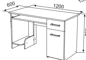
Masă calculator Star
