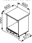
MI 2 Modul inferior cuptor
